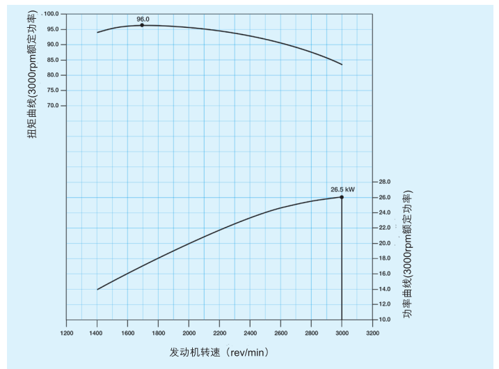
备注: 此曲线并未显示较低转速时的额定功率。
